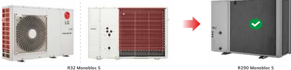
R32 Monobloc S
